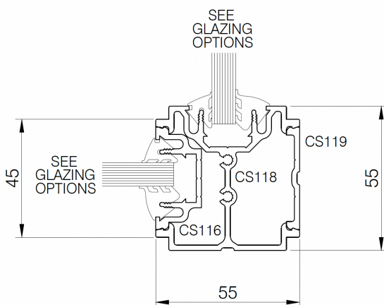
Jamb/Mullion Door Details
