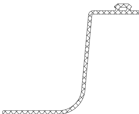
XX6013 EPDM Membrane
