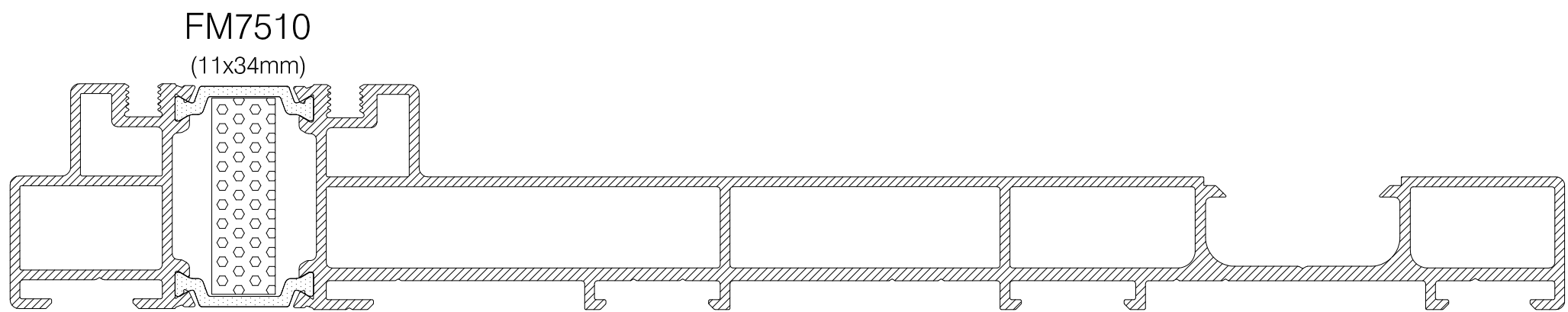
CS7519 TRIPLE DOOR JAMB
