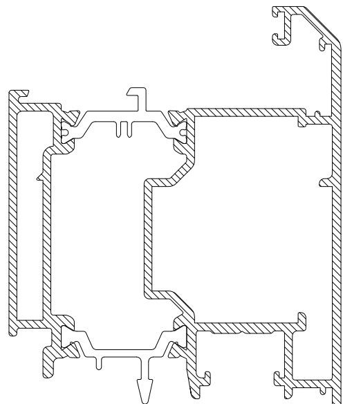
CS861 ECO DOOR LEAF OPEN OUT
