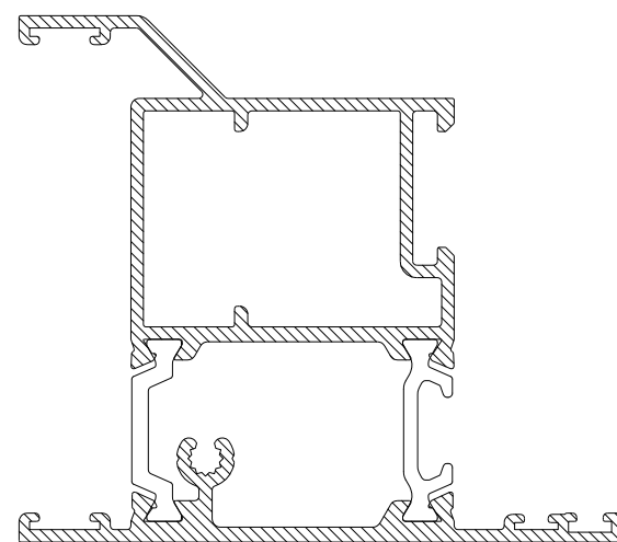
CS5868 64mm DOOR OUTER FRAME
