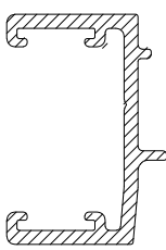
CS7210 CURTAIN WALL ADAPTOR
