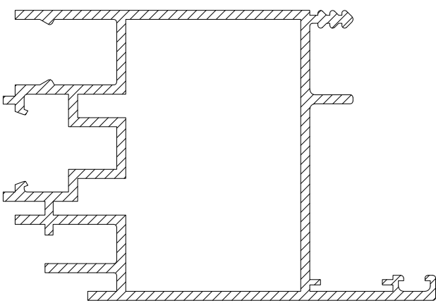
AT220 DOOR VENT FRAME
