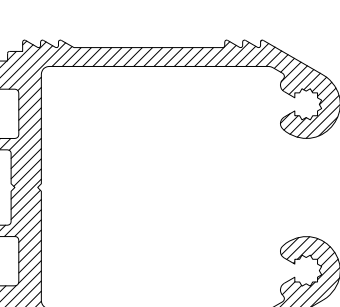
CS735 DOOR SASH SCREW TIE-ROD CLEAT
