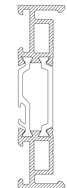
CS7004 ADJUSTABLE JAMB PART A
