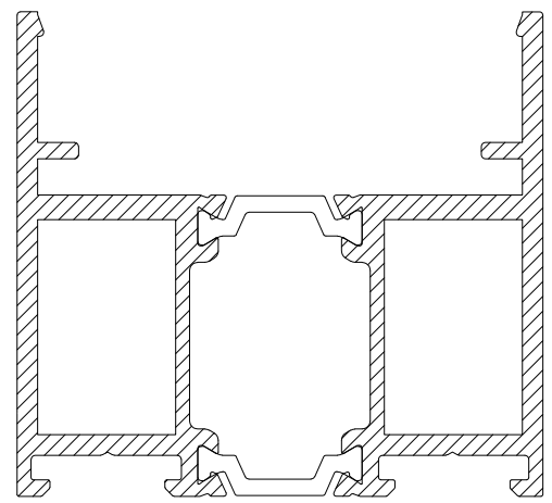
CS777 DOOR TOP RAIL
