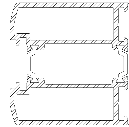
CS772 DOOR STILE, PLAIN
