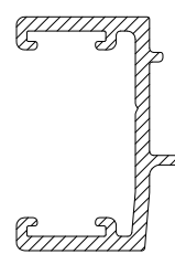
CS7210 CURTAIN WALL INSERT
