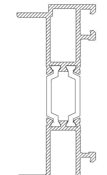
CS7005 ADJUSTABLE JAMB PART B
