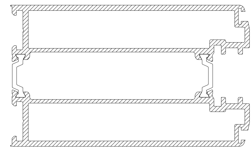
CS775 DOOR STILE WOOLPILE
