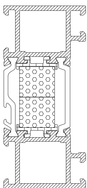
CS7001 35mm FIXED JAMB
