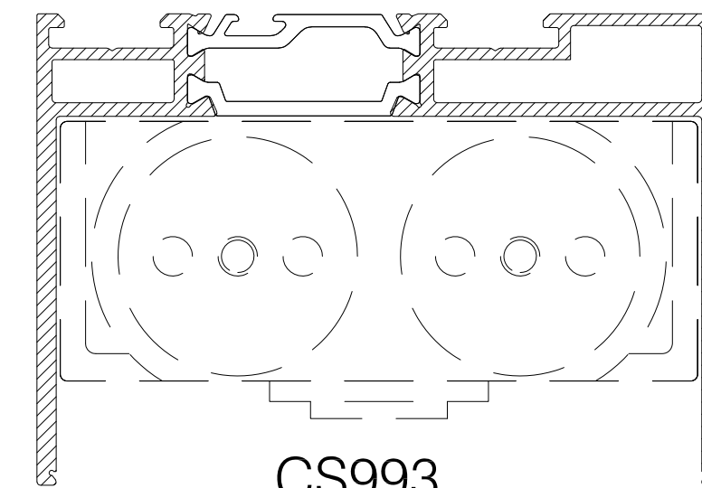
CS993 HEADER BAR
