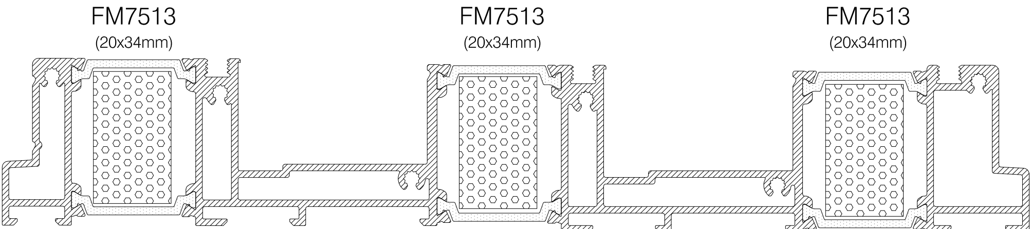
CS7518 TRIPLE DOOR FRAME
