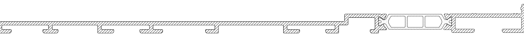
CS7521 TRIPLE DOOR SUB SILL
