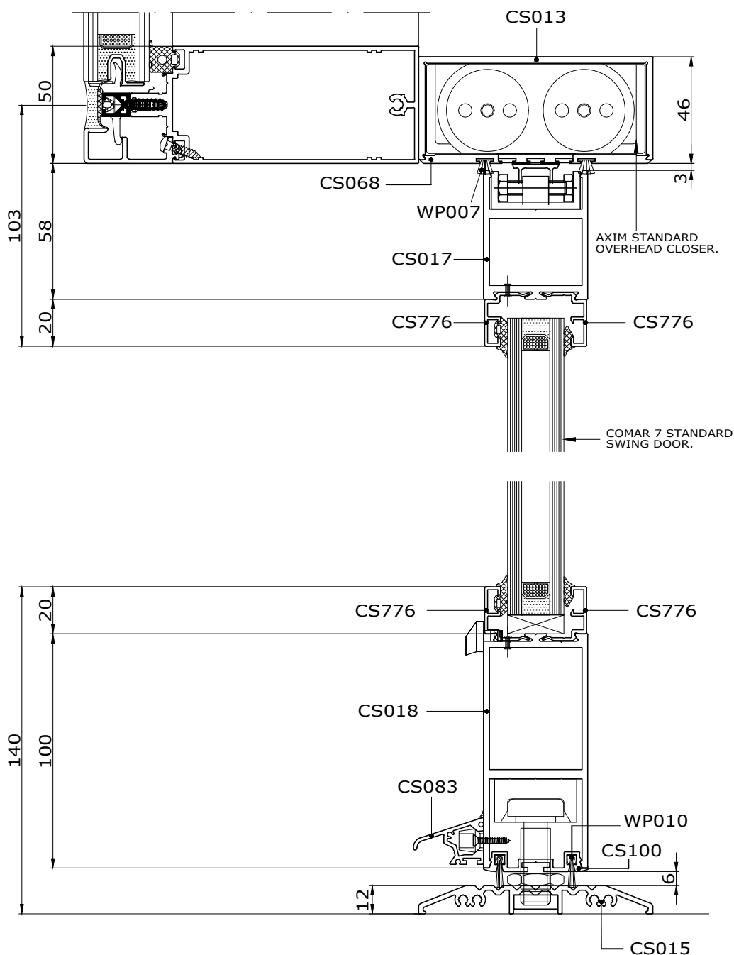
SECTION A-A
