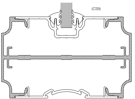
CS71 DOOR FRAME (FINGER GUARD)
