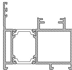
CS762 INWARD OPENING DOOR OUTER FRAME
