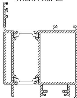
CS763 INWARD OPENING DOOR LEAF
