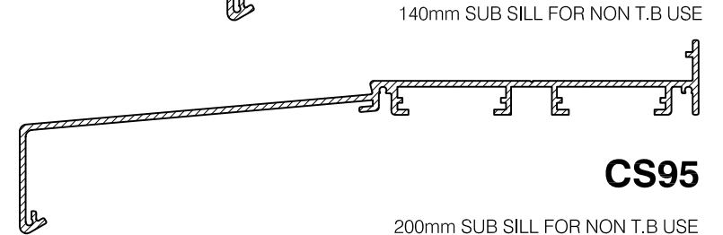
CS41R 140mm SUB SILL FOR NON T.B USE
